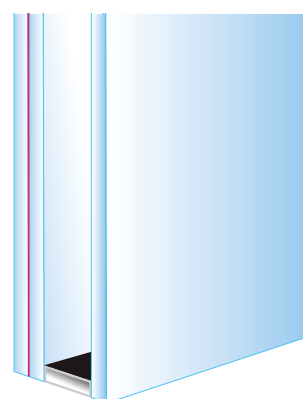
Vitrage classe 5 10P5/-/4 (10P5 correspond à 44°)
