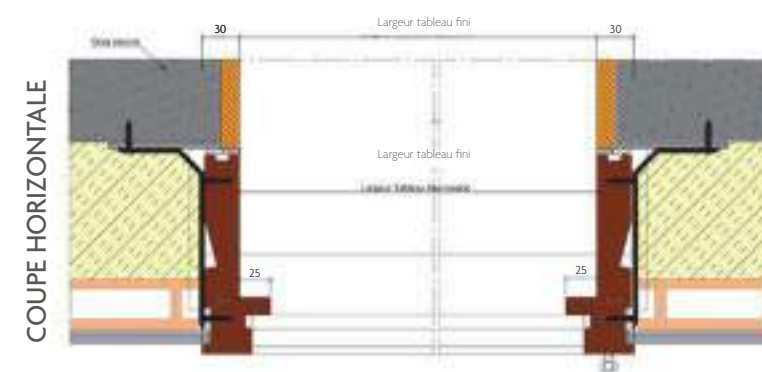
Prise de cotes largeur La mesure s'effectue à l'extérieur entre les 2 montants de la maçonnerie finie.
